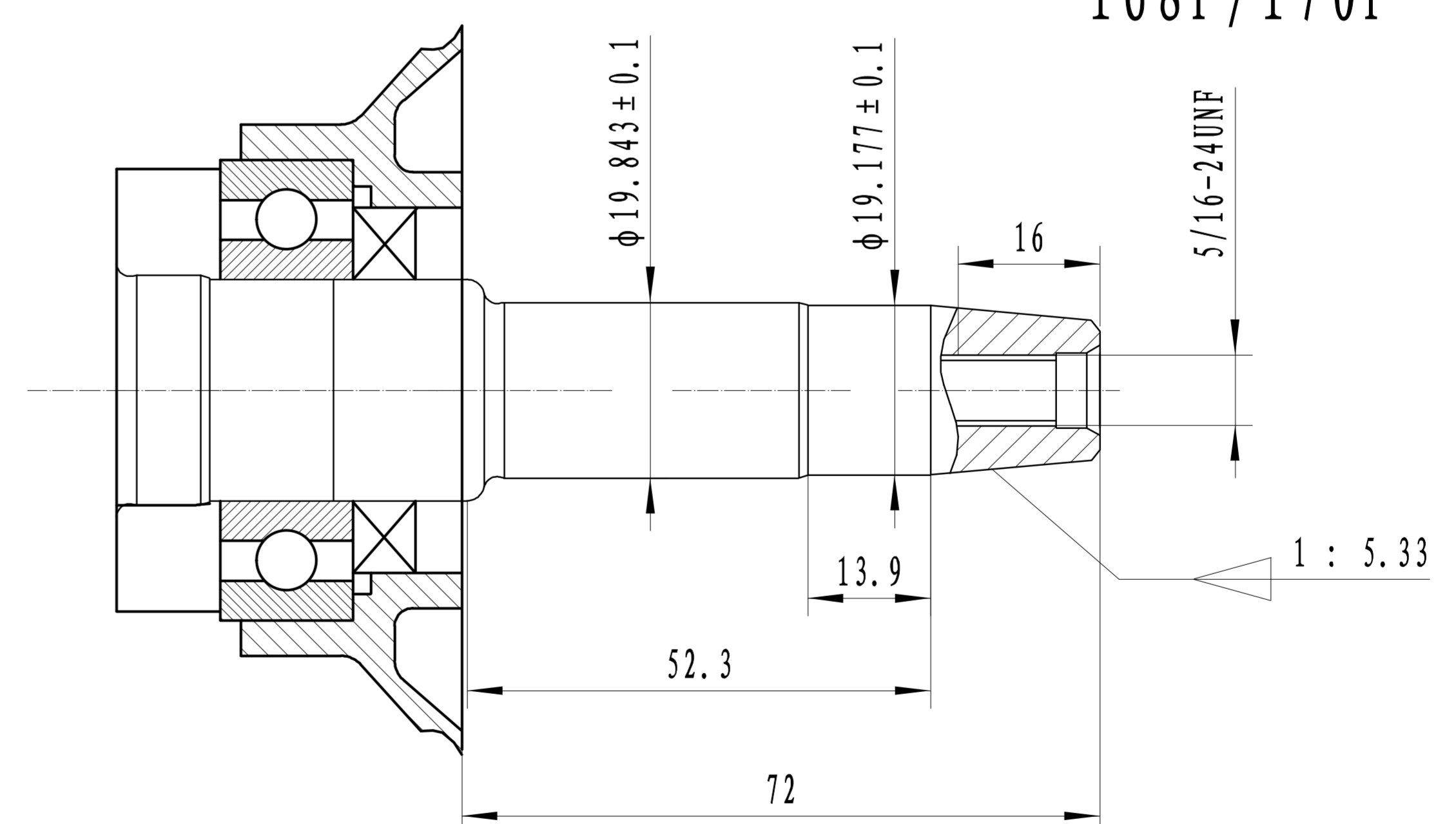
168F/170F V轴
