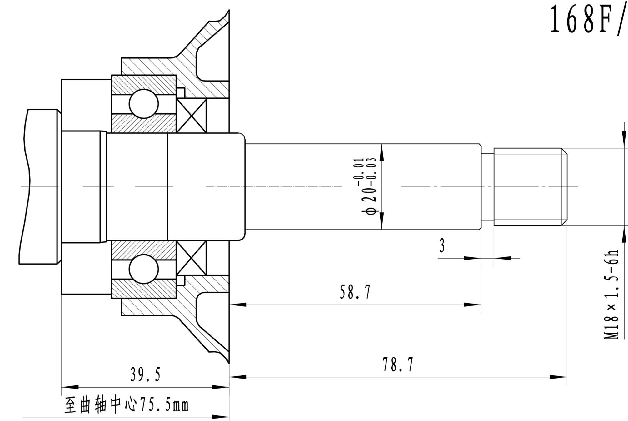
168F/170F V轴
