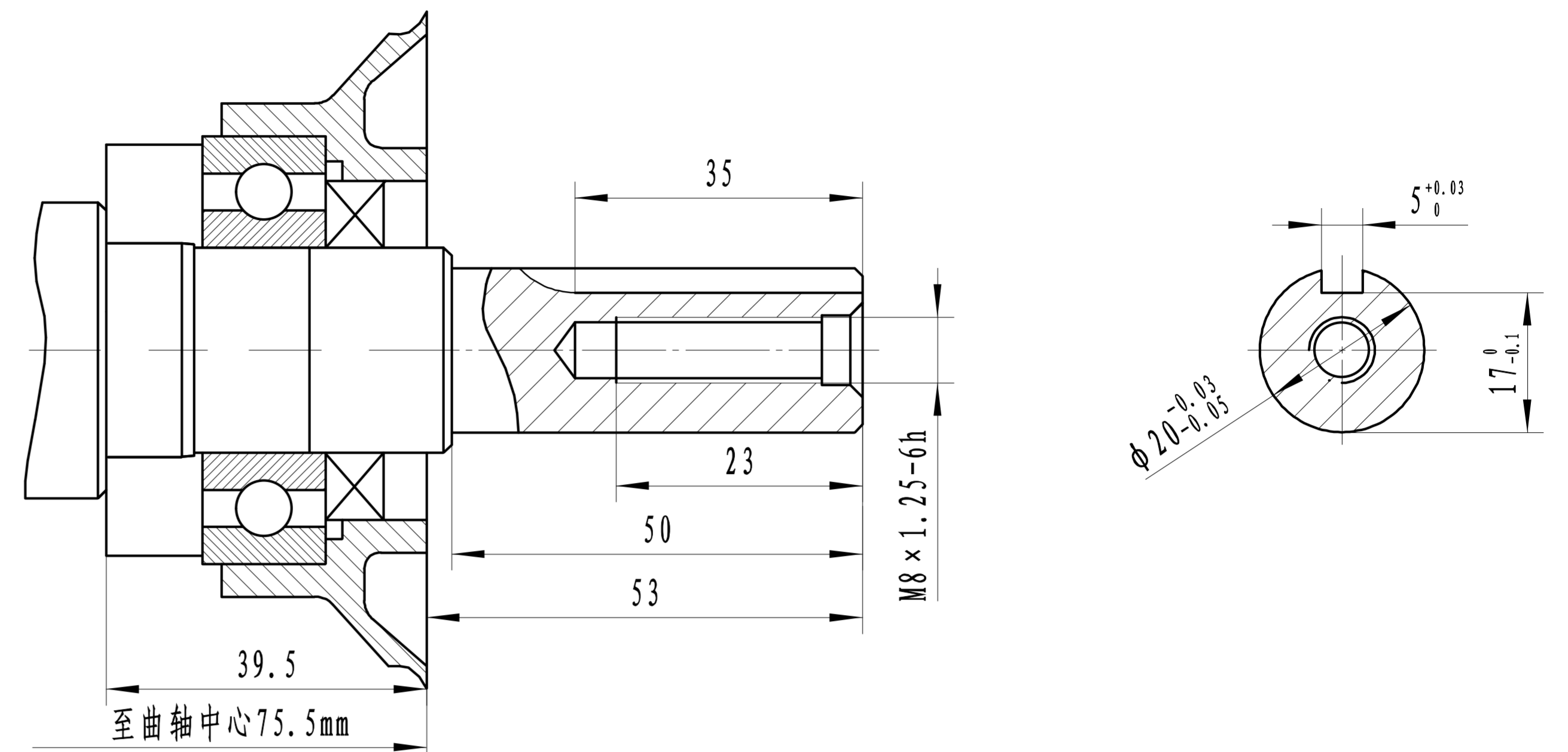
168F/170F P轴
