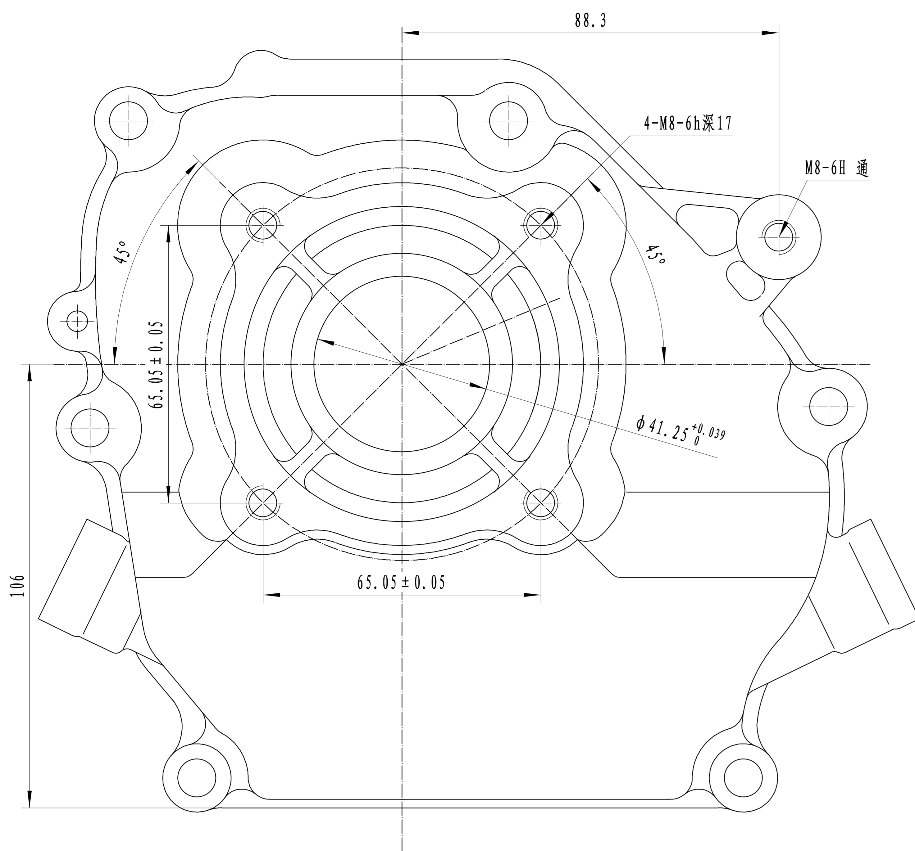
168F/170F 动力盖
