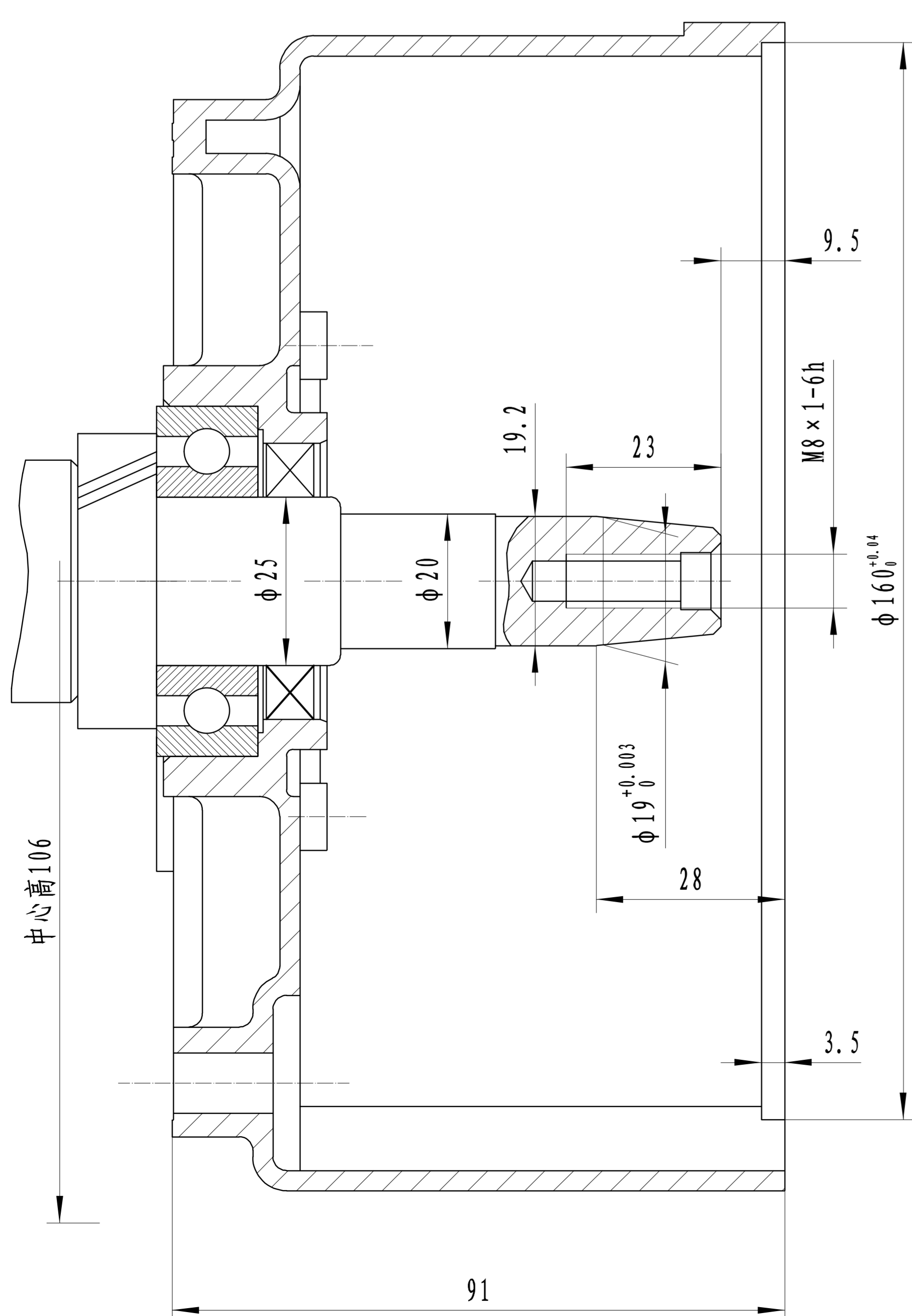
168F/170F 电机轴
