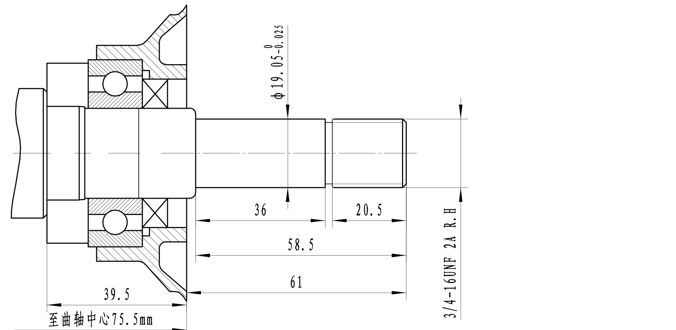
168F/170F W轴
