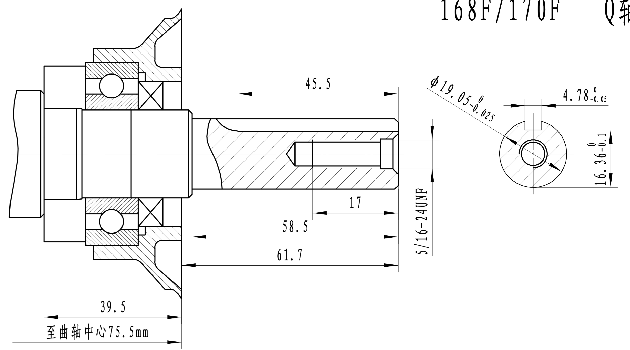
168F/170F S轴
